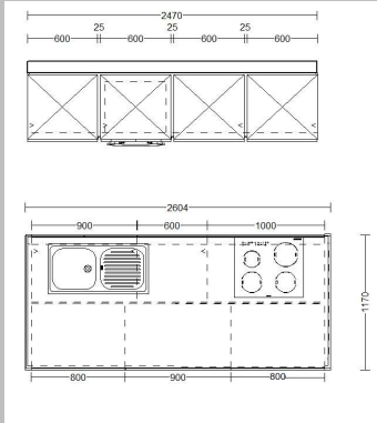
Grundriss
