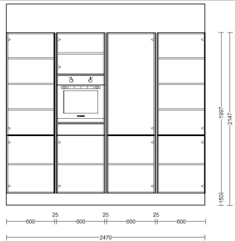
Wandansicht 1
